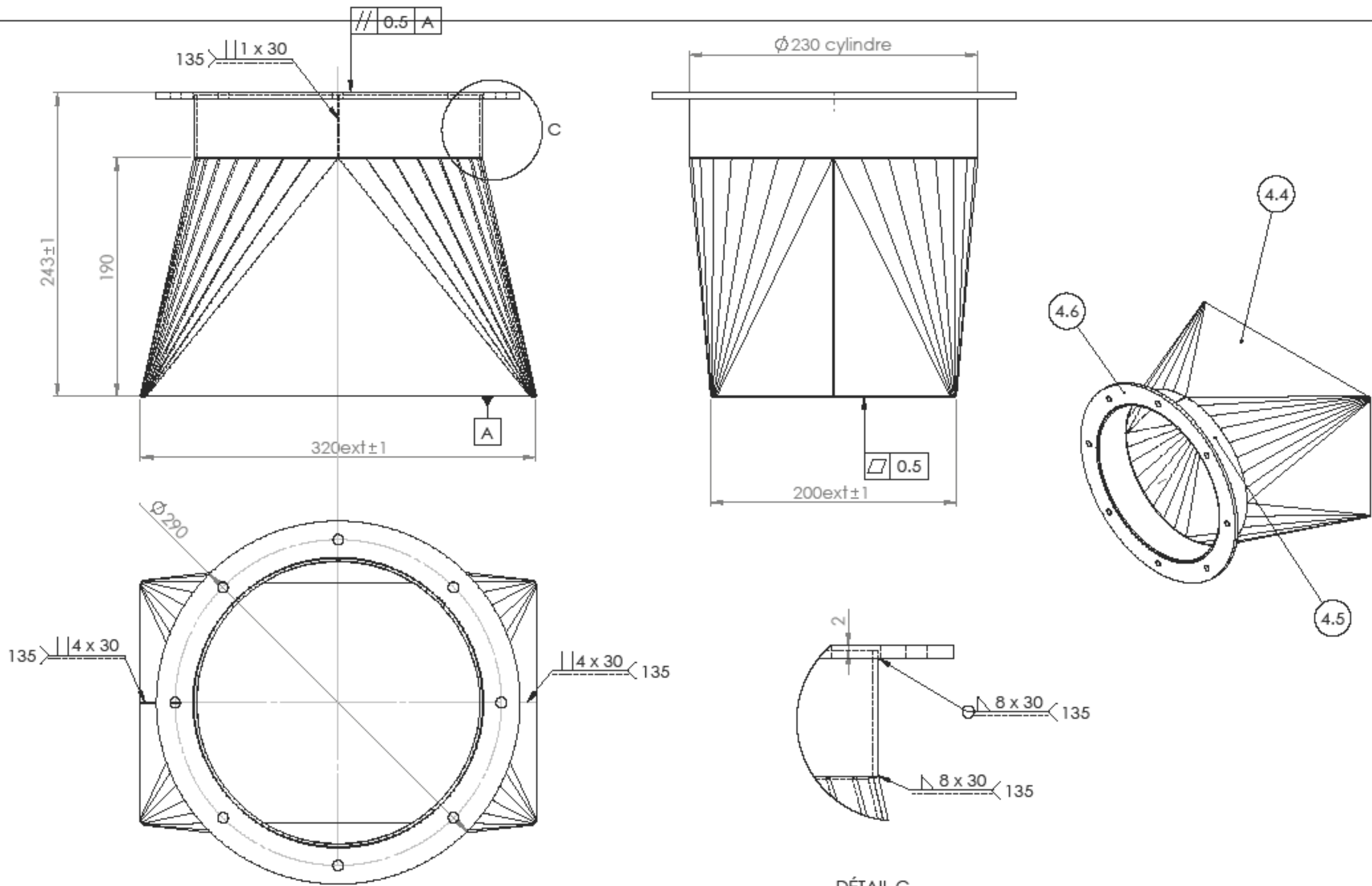
DÉTAIL C ECHELLE 2 : 3
